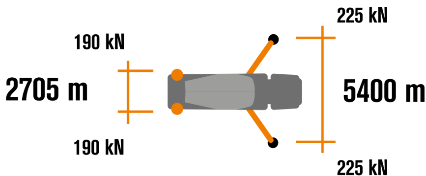
Abbildung 2: Grundfläche Abstützung - Quelle Prospekt CIFA MK28L
