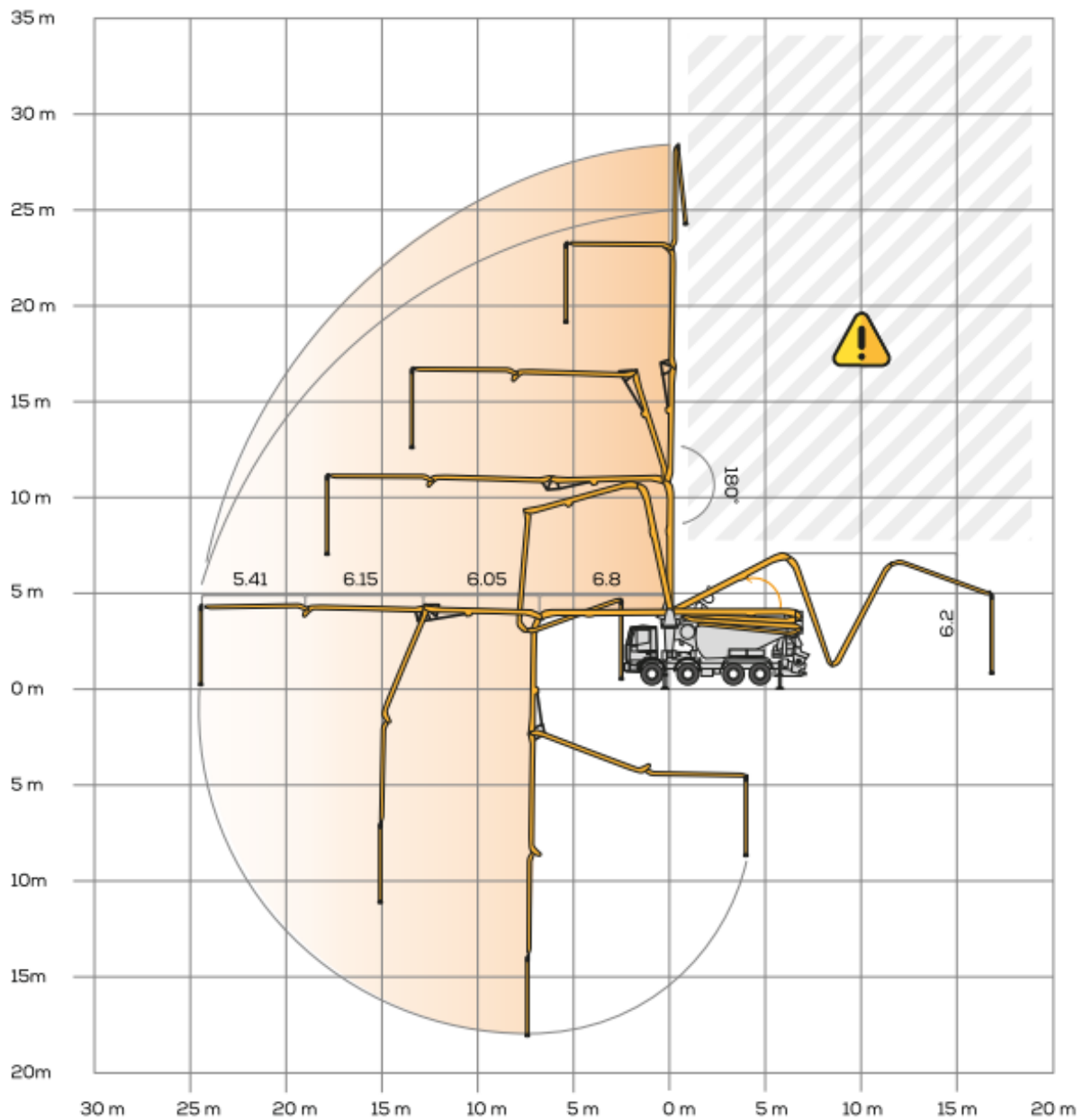
Abbildung 3: Reichweite Ausleger - Quelle Prospekt CIFA MK28L
